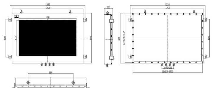
加固智控大屏外形示意图
